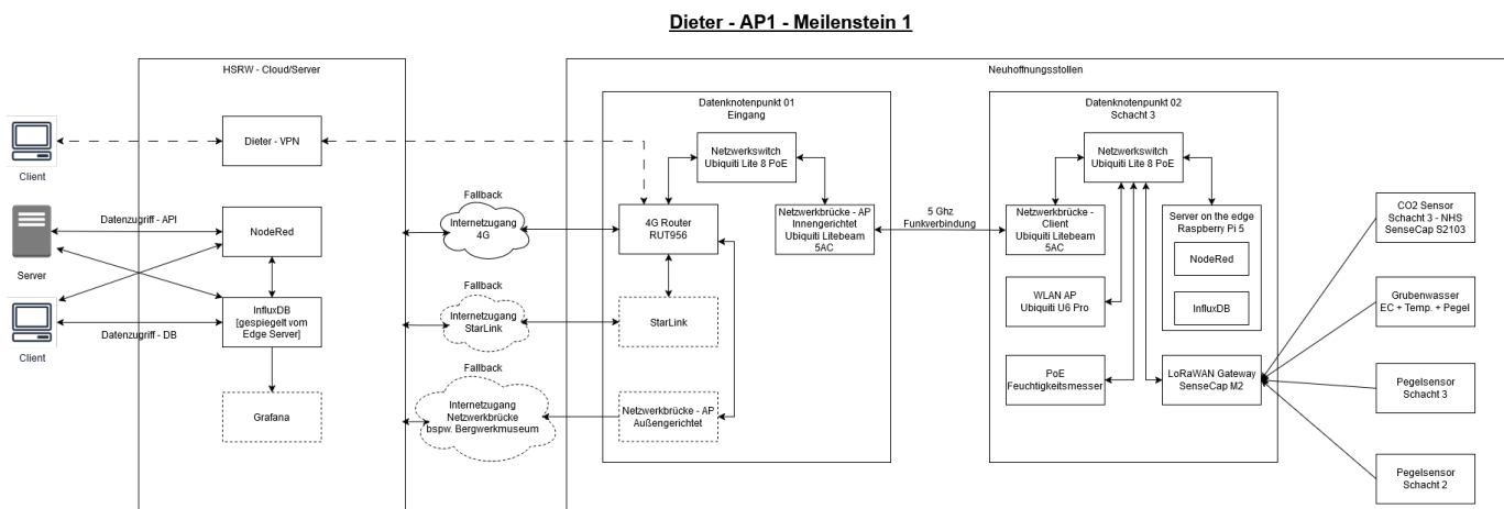
Fig. 2: Netzplan - Neuhoftungsstollen in Bad Ems - Stand: 14.01.2025 Innerhalb des Stollens arbeiten wir mit Datenknotenpunkten (DKP). Der wichtigste Ort hier im Projekt ist der Raum um den Schacht Nummer 3. Hier befindet sich der Hauptknotenpunkt des Netzwerks. Dieser beinhaltet den Server und auch das LoRaWAN Gateway inkl. des Netzwerk-Servers der dafür benötigt wird. Die Verbindung zwischen den beiden DKPs wird über eine Richtfunkstrecke, welche im 5 Ghz Bereich funkt hergestellt. Der Cloud-Server wird von der HSRW bei Netcup gehostet, da die Dienste lediglich gering ausgelastet sind, da nur ein Stollen momentan versorgt wird, reicht bereits ein sehr kleiner V- oder Root-Server aus, welcher im Monat nur geringe Kosten verursacht. Durch entsprechende Konfiguration ist es so auch möglich auf die Geräte und Dienste, welche auf dem Server im Bergwerk installiert sind, zuzugreifen.
