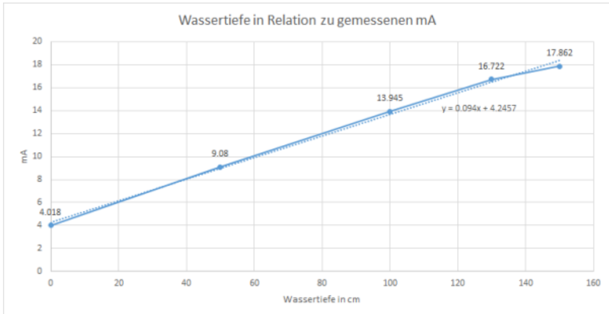
Fig. 1: Umrechnung von mA zu cm
